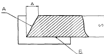
Рисунок 1. Отклонение торца проката от перпендикулярности
